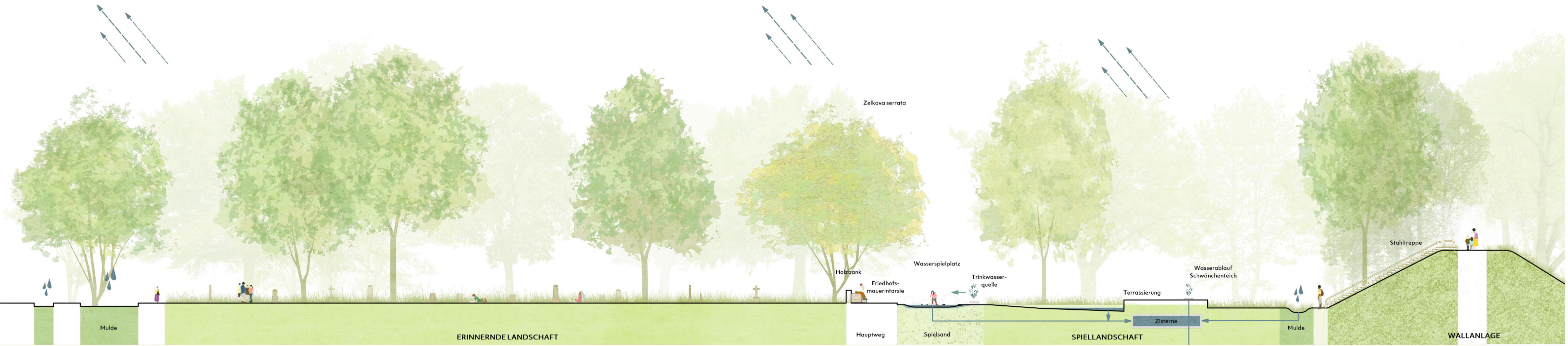
Geländeschnitt 2 Süd 1:200
