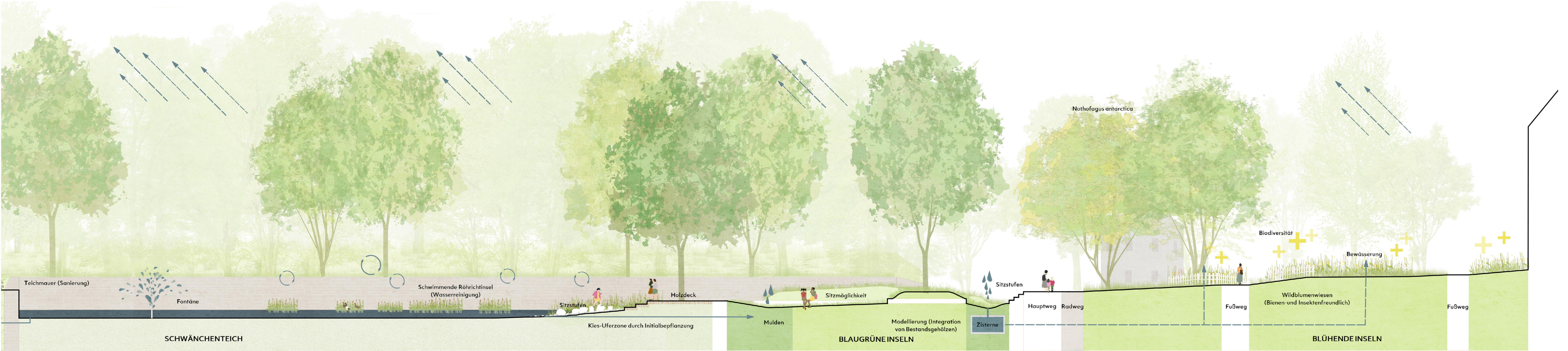
Geländeschnitt 1 Nord 1:200
