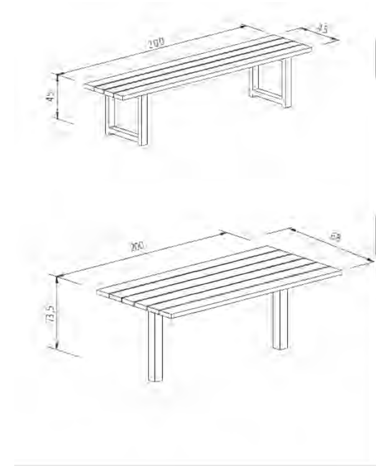
Variante Tisch und Hockerbank, Bank Lagarda
