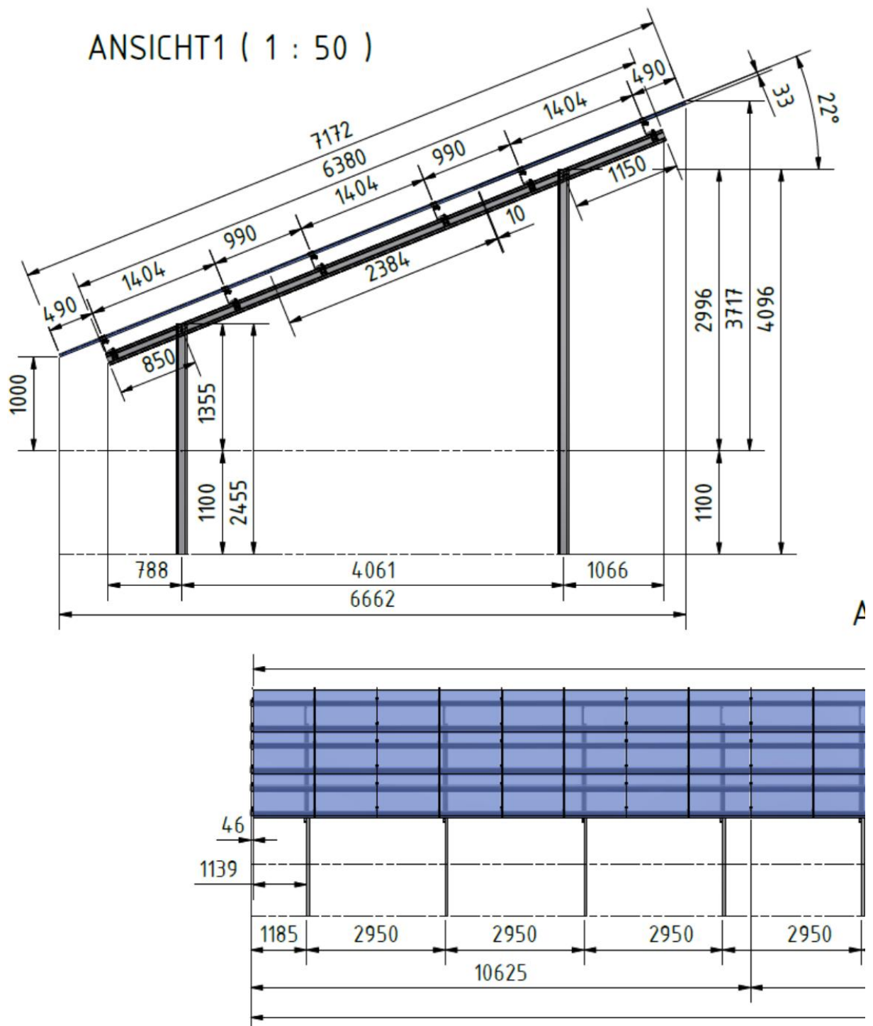
Abb. 3: Typische Abmessungen des Ständerwerkes für PV-Modultische (hier: PV-Anlage Deiderode der Stadtwerke Göttingen AG).
