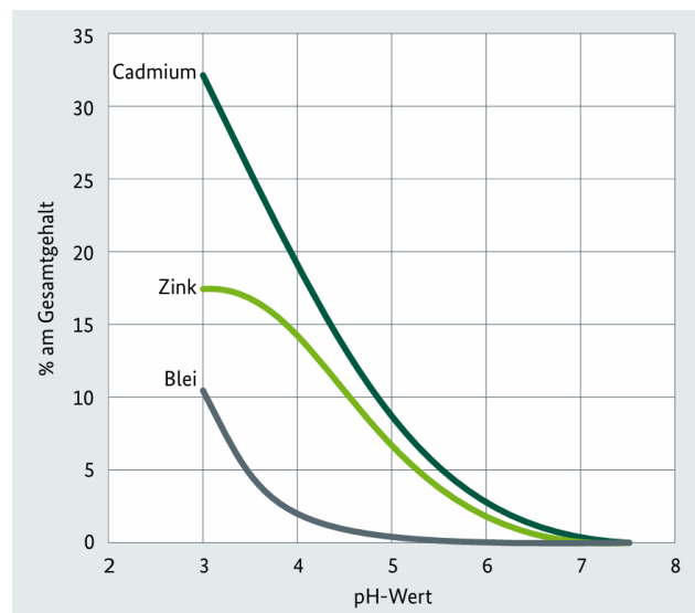
Abb. 1: Pflanzenverfügbare Schwermetallgehalte (in Prozent der Gesamtgehalte) in Abhängigkeit vom pH-Wert (Quelle: Bundesanstalt für Landwirtschaft und Ernährung 8 )
