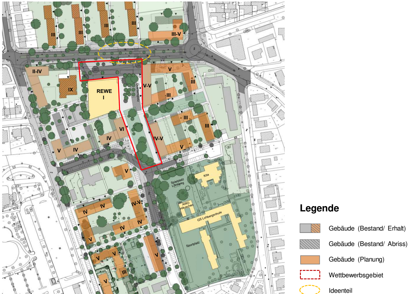
Rahmenplan „Grüne Mitte Ebertal“ mit Markierung des Wettbewerbsgebiets (Darstellung: Stadt Göttingen)
