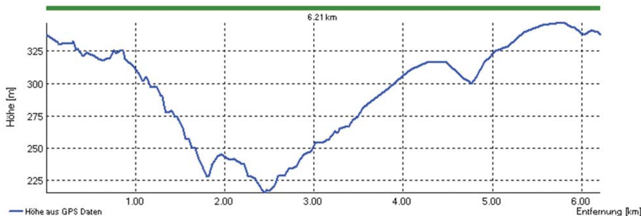
Höhenprofil
