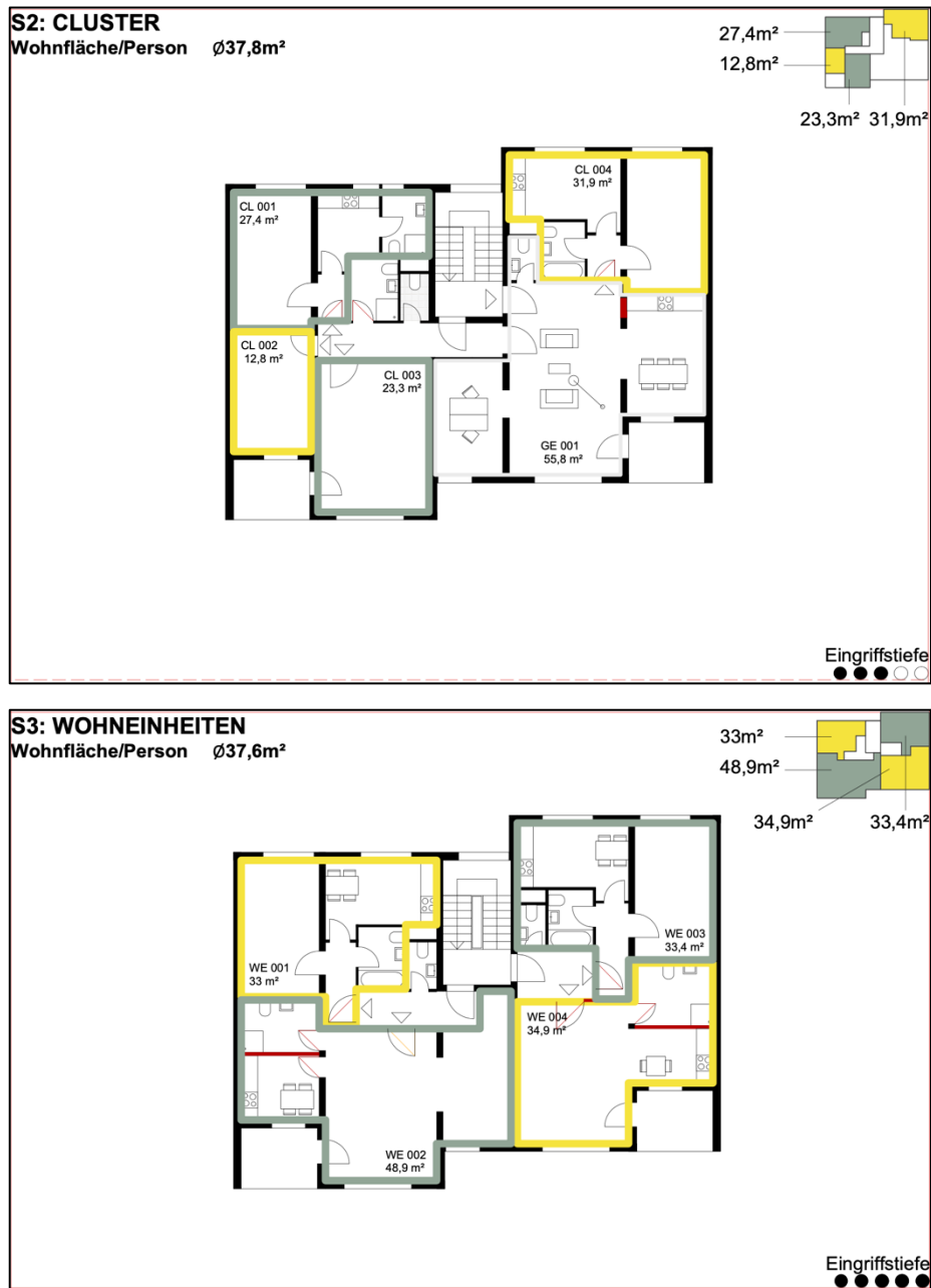
Abbildung 5 Grundrisstyp eines Mehrfamilienhauses und Darstellung der möglichen Teilbarkeit, Umwandlung in eine Clusterwohnung und Nutzbarkeit als Wohngemeinschaft
