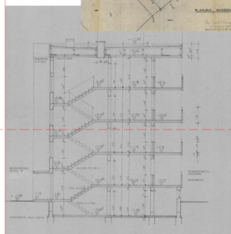
Abb.X: Schnitt Süd-Ost V_1Sp_M; Bestandspläne Hofheimer Wohnungsbau GmbH
